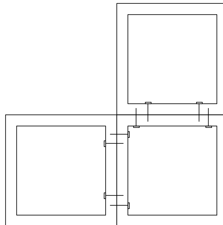
Detalle Encuentros
